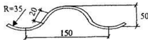
Рис. П.1.3. Профиль гофрированного листа:
