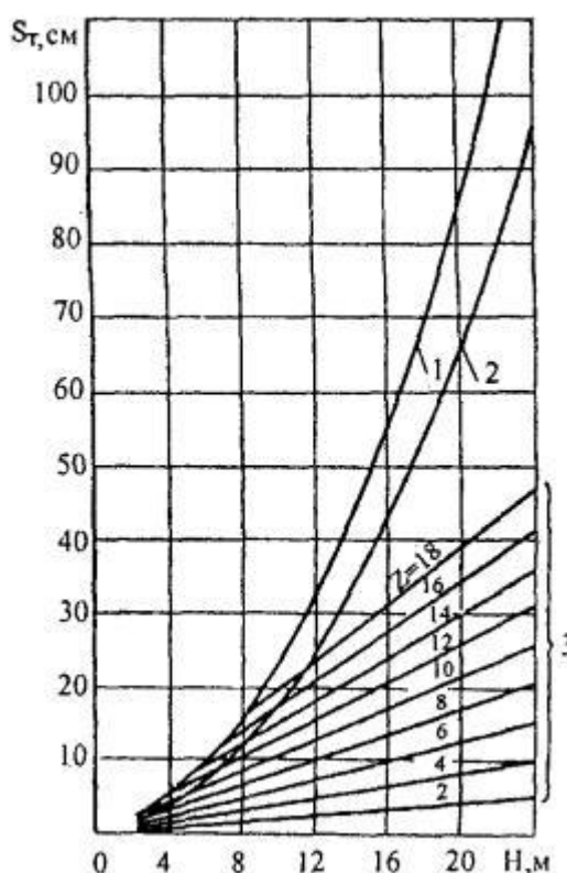
Рис. П.6.1. Расчетный график для определения осадки трубы:
