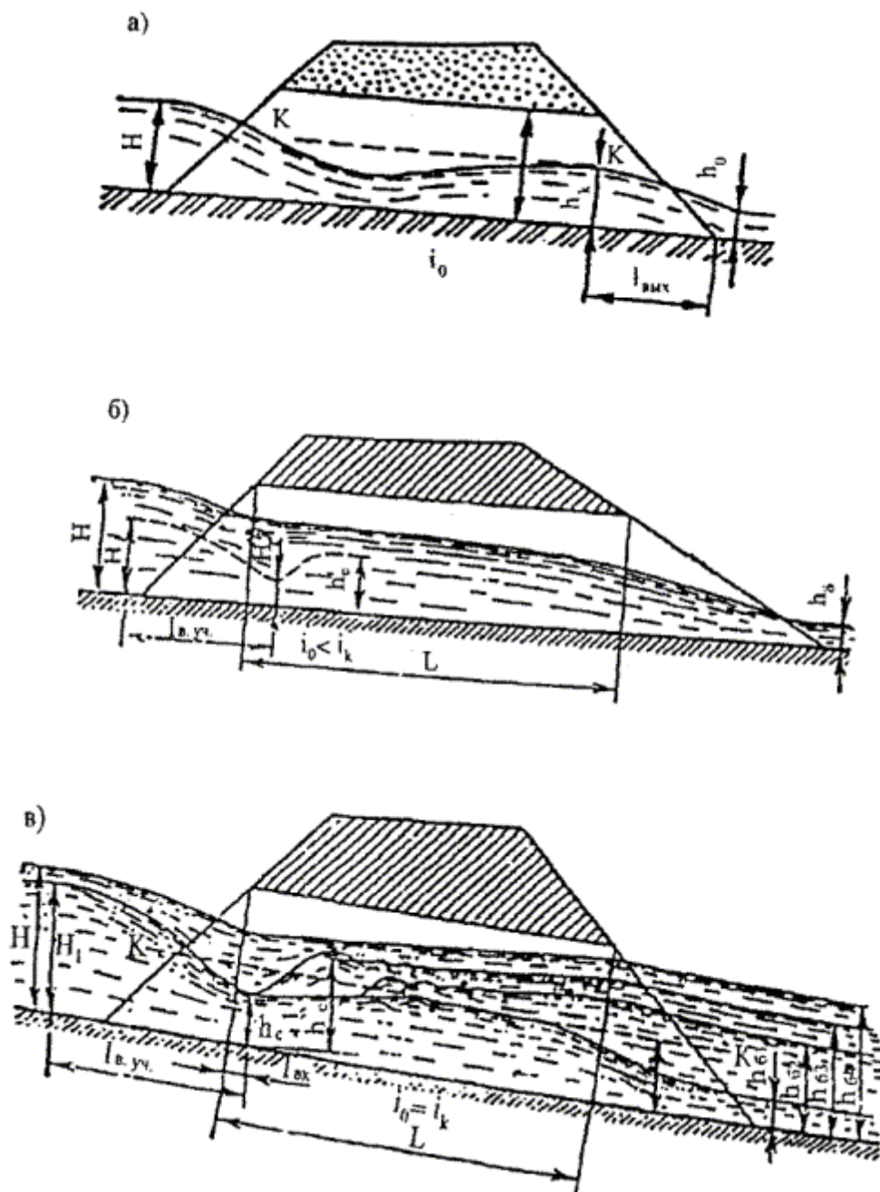
Рис. П.3.1. Схема протекания воды в равнинной трубе при безнапорном режиме:
