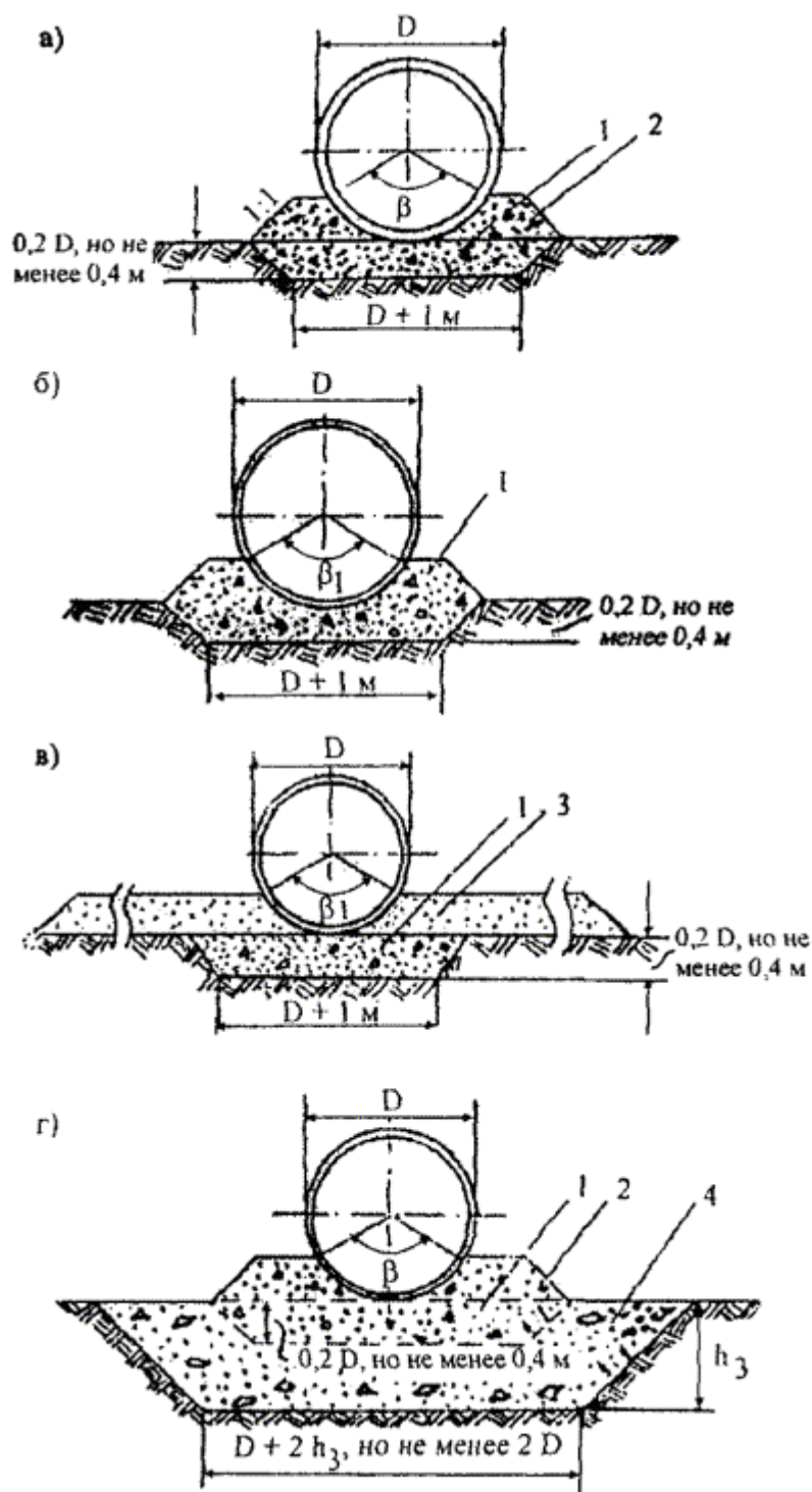
Рис. 2. Конструкция основания под трубами:
