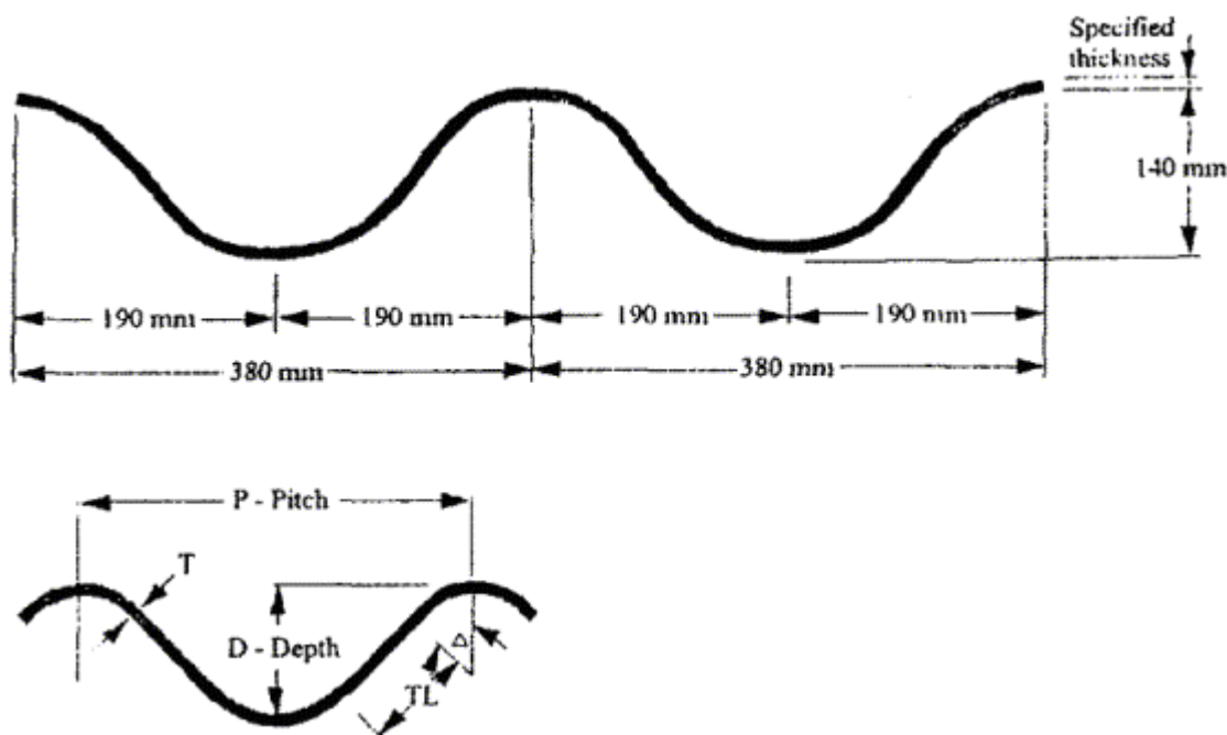
Рис. П.1.4. Профиль гофрированного листа:
