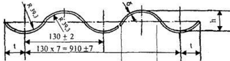
Рис. П.1.1. Профиль гофрированного листа:
