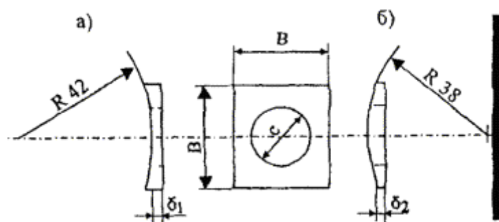
Рис. П.2.1. Шайбы для болтов (размеры в миллиметрах):
