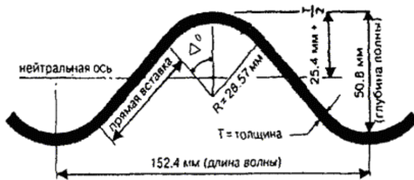
Рис. П.1.2. Профиль гофрированного листа:
