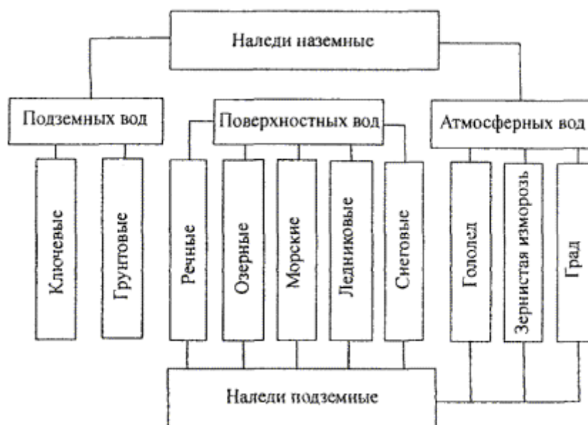
Рис. 1. Схема классификации наледей (по Алексеву, Савко, 1975)
